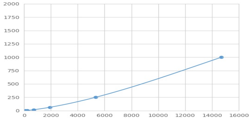
(甘氨酸tRNA合成酶)检测试剂盒标准曲线
