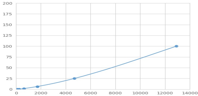
(唾液富组蛋白3)检测试剂盒标准曲线
