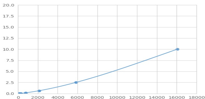
(亨廷顿蛋白)检测试剂盒标准曲线
