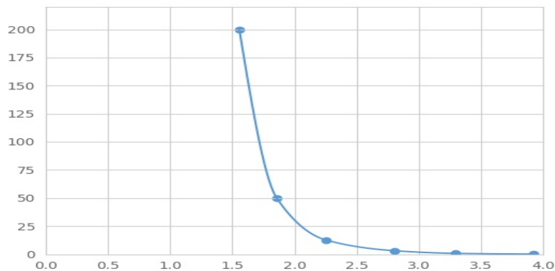
(吲哚乙酸) 检测试剂盒标准曲线
