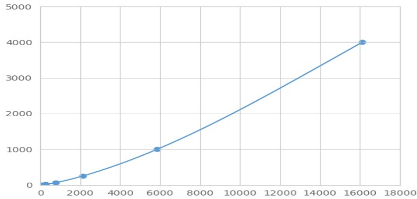
(胰岛素样生长因子结合蛋白7)检测试剂盒标准曲线
