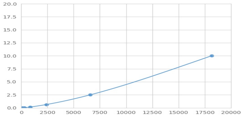
(整合素 \alpha 9) 检测试剂盒标准曲线
