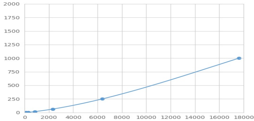
(淋巴毒素β)检测试剂盒标准曲线
