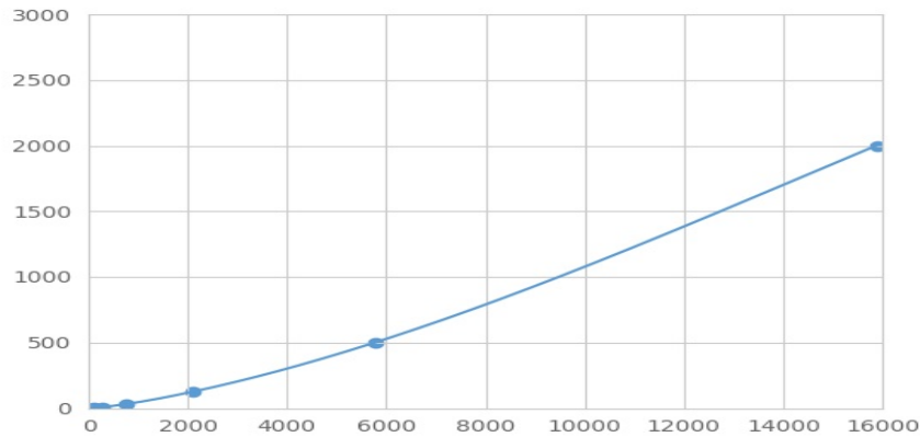
(甘露糖苷酶 α 2B类成员1)检测试剂盒标准曲线
