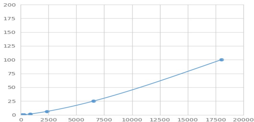
(脑膜瘤表达抗原5) 检测试剂盒标准曲线
