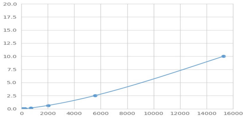
(髓鞘碱性蛋白)检测试剂盒标准曲线
