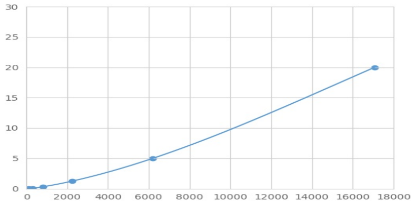
(NK6同源框蛋白1)检测试剂盒标准曲线
