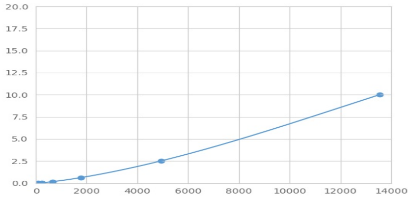
(外周蛋白)检测试剂盒标准曲线
