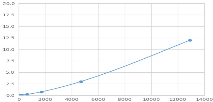
(IIA组磷脂酶A2) 检测试剂盒标准曲线
