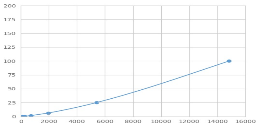
(磷脂酶D2) 检测试剂盒标准曲线
