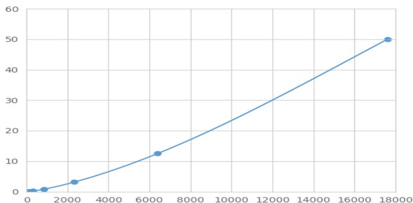
(唾液淀粉酶 \alpha 1)检测试剂盒标准曲线
