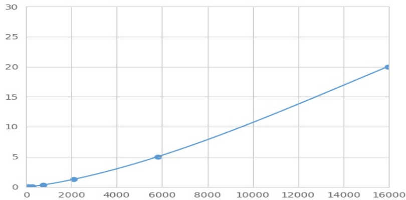
(突触囊泡蛋白VII)检测试剂盒标准曲线
