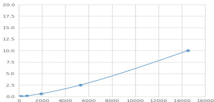
(味觉受体1型成员2)检测试剂盒标准曲线
