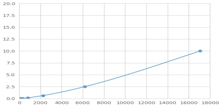
(转录因子7样蛋白2)检测试剂盒标准曲线
