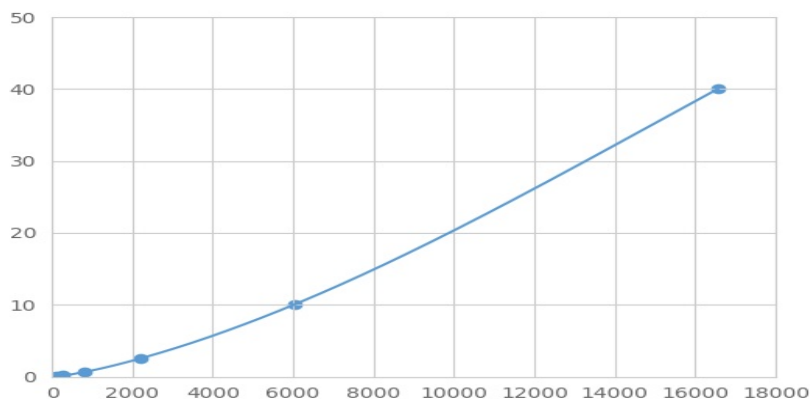
(丙糖磷酸异构酶1) 检测试剂盒标准曲线
