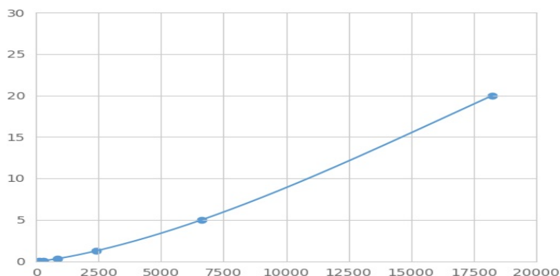
(泛素A52残留核糖体蛋白融合产物1)检测试剂盒标准曲线
