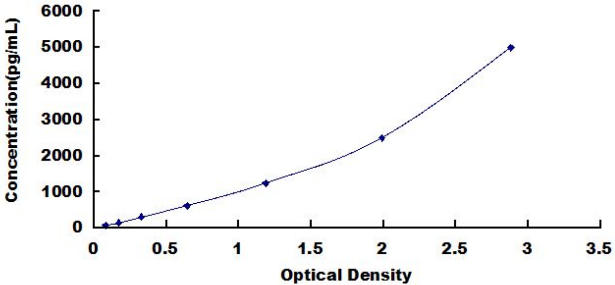
小鼠趋化因子 C-X3-C-基元配体 1 (CX3CL1) 检测试剂盒标准曲线
