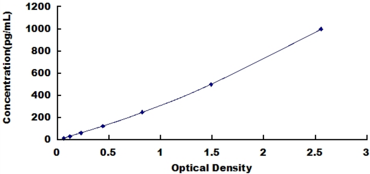
人粒细胞集落刺激因子 (G-CSF) 检测试剂盒标准曲线
